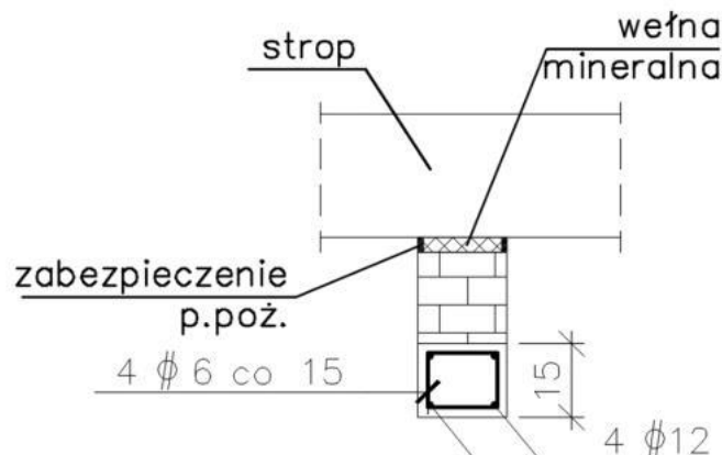
Rys. nr 2 Schemat wykonania nadproża żelbetowego.
