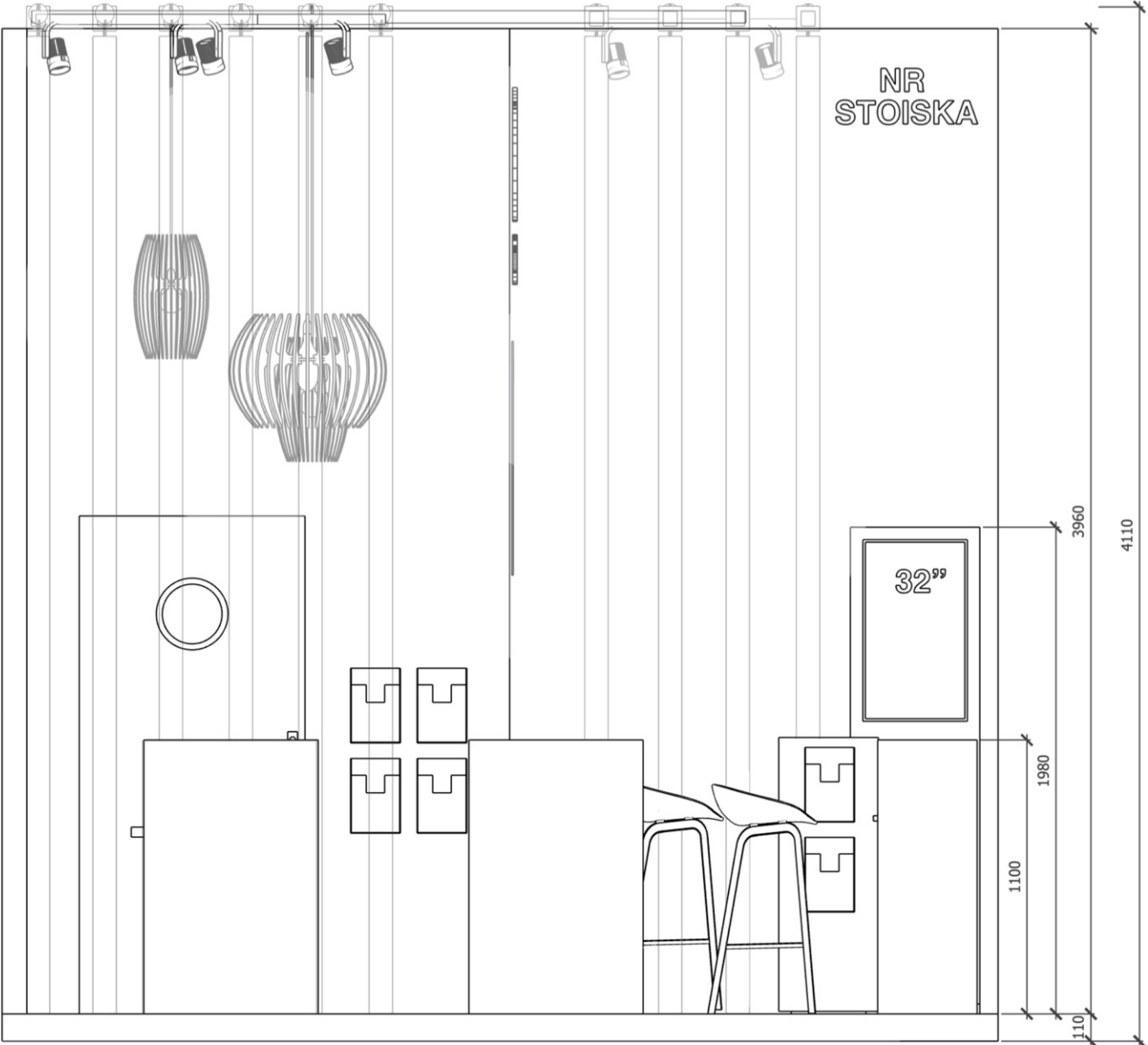
WIDOK A-A
