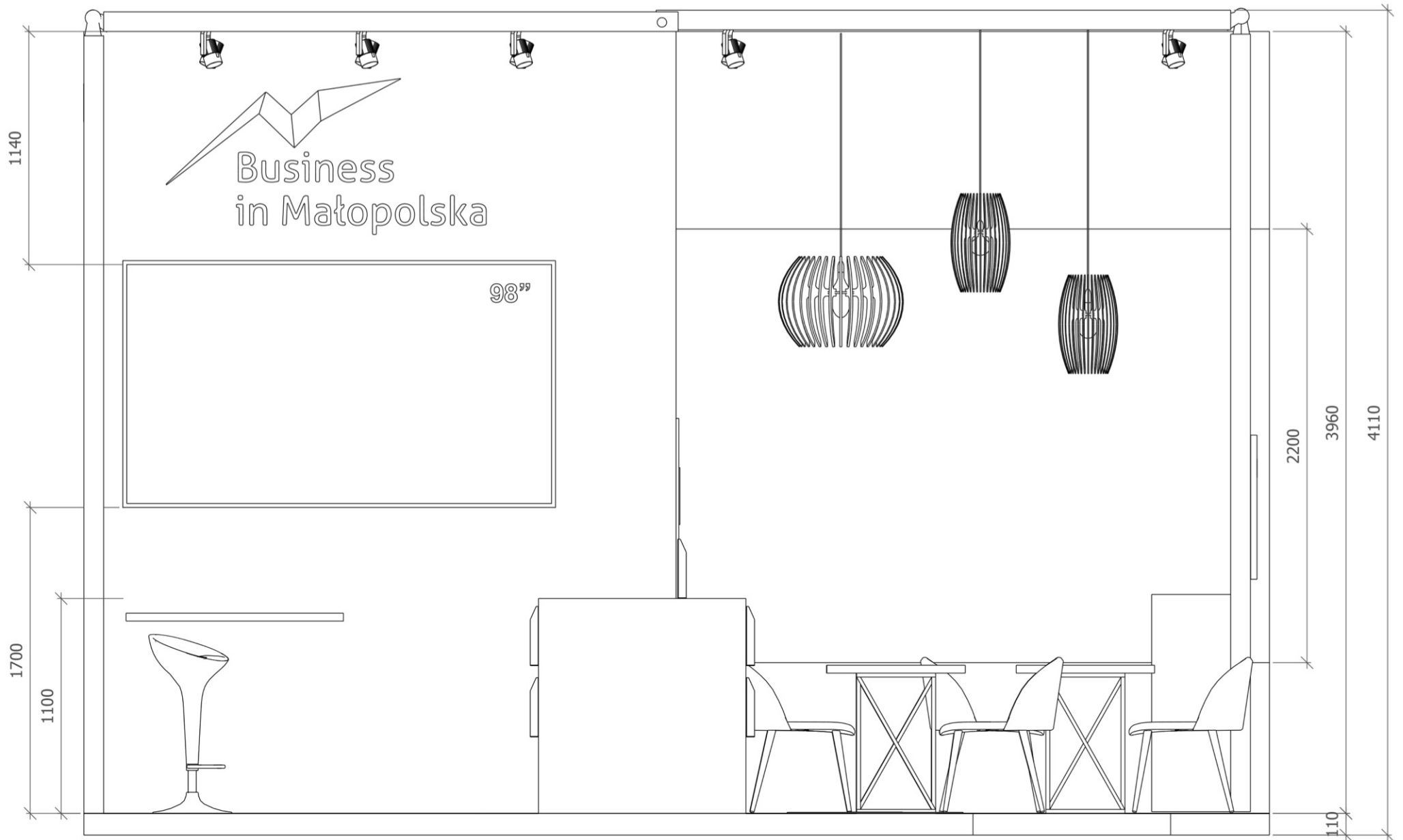
WIDOK B-B
