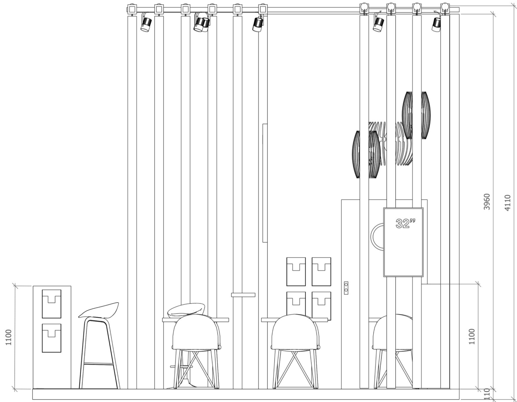
WIDOK A-A
